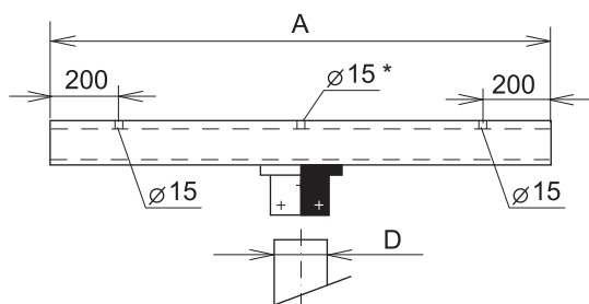
KONZOLE PRO REFLEKTORY CONSOLE FOR SPOTLIGHTS
