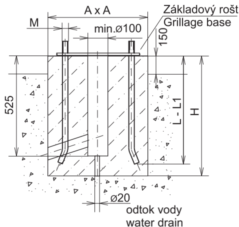
KOTVENÍ K ZÁKLADOVÉMU ROŠTU GRILLAGE BASE ANCHORING
