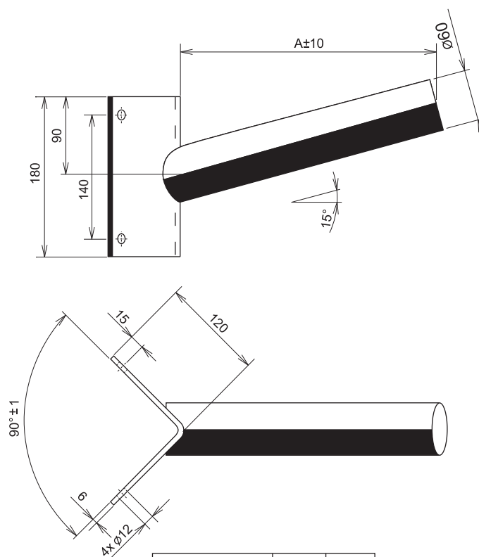
NÁSTĚNNÁ ROHOVÁ KONZOLE CORNER WALL CONSOLE
