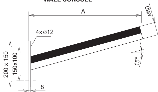
NÁSTĚNNÁ KONZOLE WALL CONSOLE
