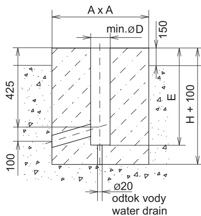
KOTVENÍ V ZEMI GROUND ANCHORING
